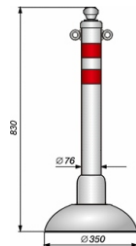
Съемный противотаранный
